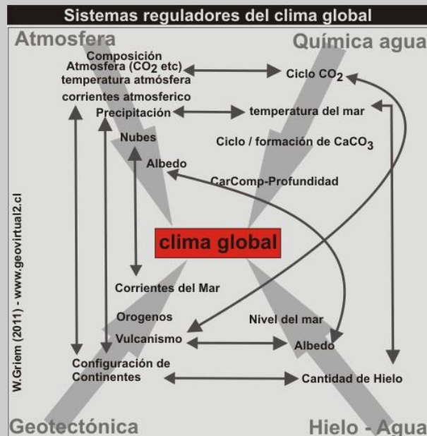
Figura: Factores del clima global. Si se propone los cuatro grandes sistemas terrestres (Agua - Hielo, Química del agua, Atmosfera y geotectónica) ya se produce un sistema de alta complejidad. Por ejemplo la acción del ser humano en los últimos 200 años altero en forma considerable la cantidad de CO 2 en la atmosfera que por cierto, afecta a muchos otros factores. En el modelo presentado arriba no se toma en consideración factores externos como cambios actividad solar o impacto de meteoritos.
