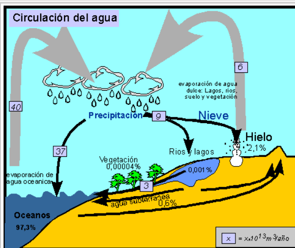
Figura: Circulación del agua: La versión simplificada, entre océanos, ríos, lagos, vegetación, hielo y atmósfera. En un modelo más avanzado hay que agregar procesos geodinámicos como la subducción y magmagenesis.
